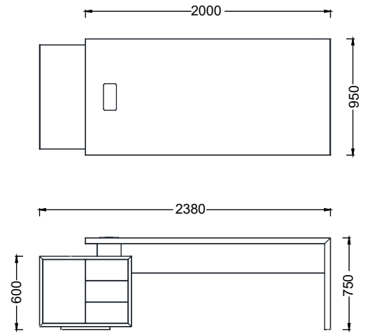
FEMO20095- YENİ FORMA SOL ETAJERLİ MASA 200X95 (Melamin)
