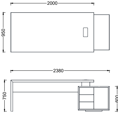
FEMA20095- YENİ FORMA SAĞ ETAJERLİ MASA 200X95 (Melamin)
