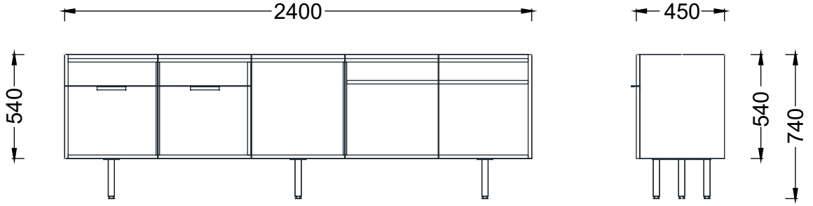
FKY24045-YENİ FORMA KONSOL (Melamin)
