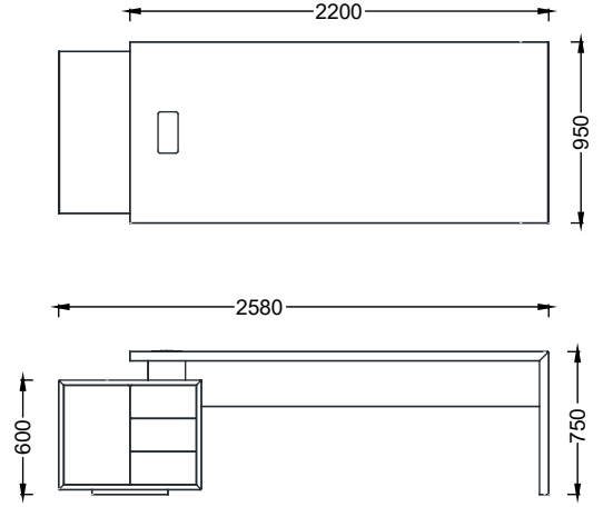
FEMO22095- YENİ FORMA SOL ETAJERLİ MASA 220X95 (Melamin)
