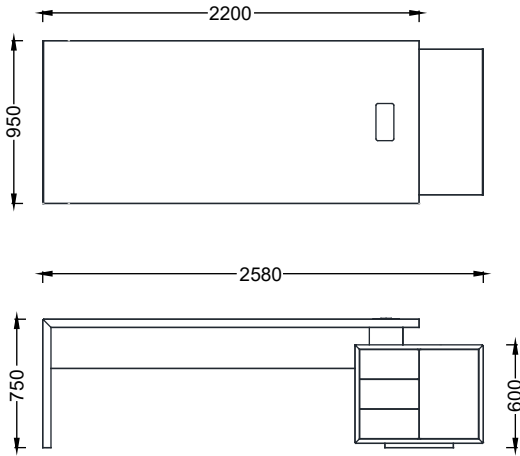
FEMA22095- YENİ FORMA SAĞ ETAJERLİ MASA 220X95 (Melamin)
